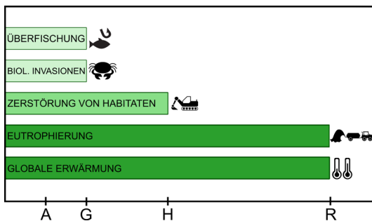
Abb. 4.11-2: Vorherrschende anthropogene Einflüsse auf die verschiedenen Ebenen und Skalen der Biodiversität der Ostsee. Abkürzungen: A= Art (Gene), G= Gemeinschaften, H= Habitate, R= Regionen. Modifiziert nach HELCOM (2009).
