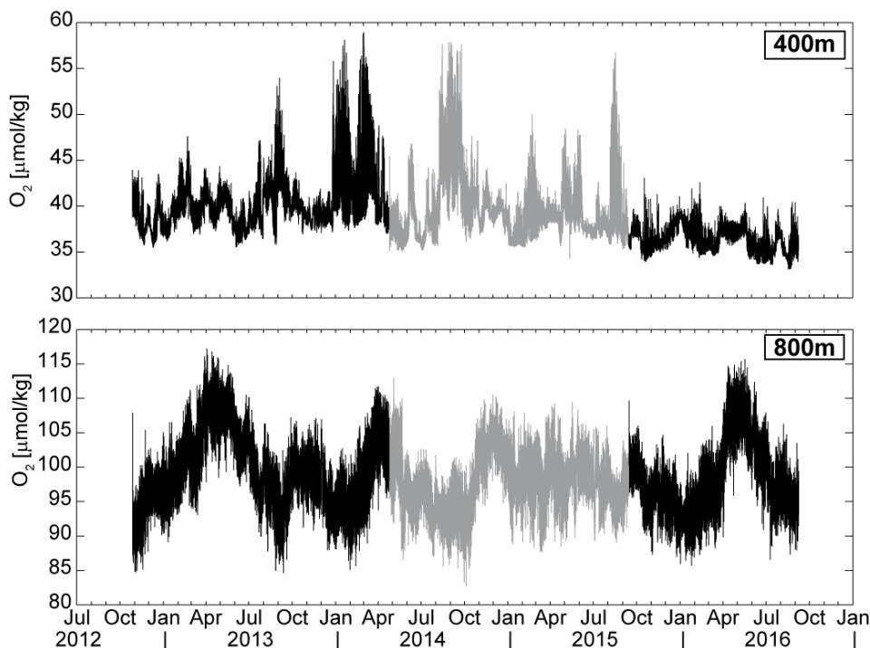
Abb. 1: Zeitserien von Sauerstoffkonzentrationen vom Zentrum der Sauerstoffminimumzone (11°N, 21°W) aus 400m (oben) und 800m (unten) Tiefe. Schwarze Linien kennzeichnen die gemessenen Konzentrationen aus der ersten (links) und der gerade abgeschlossenen dritten Auslegungsperiode (rechts). Die graue Linie kennzeichnet die Messungen der zweiten Verankerungsauslegung. (Bild: Johannes Hahn)
