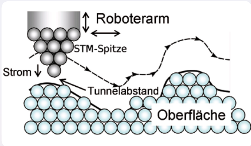
Abb. 2: Funktionsweise eines Rastertunnelmikroskops.
