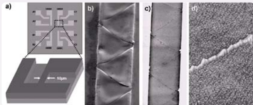
Abb. 11: Die Risse in der Oberfläche werden extra hergestellt. Sie werden mit Metall ausgefüllt, so entsteht ein Nanodraht.
