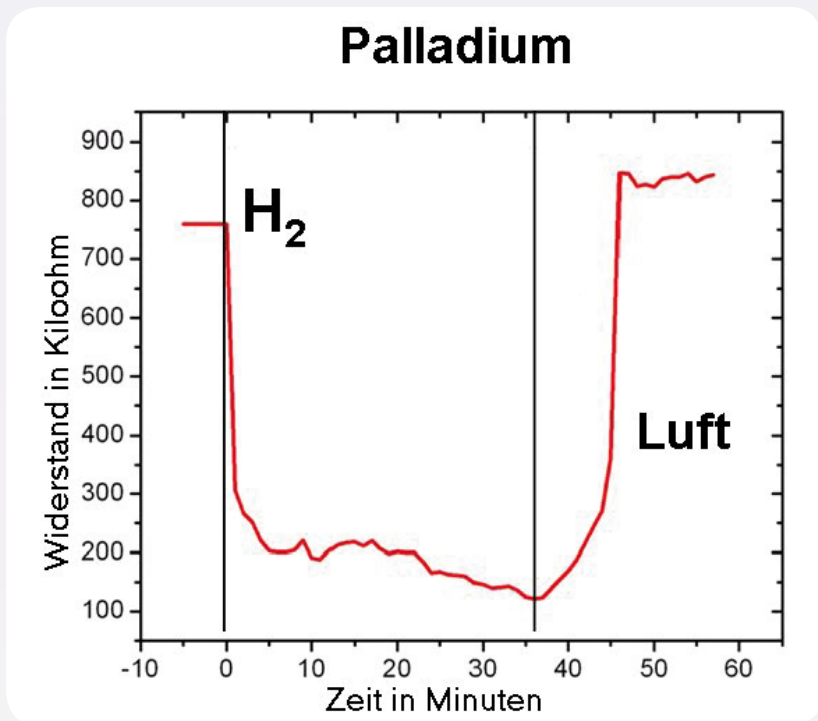
Abb. 12: Verlauf eines Empfindlichkeitsversuches: Wird der Nanodraht aus Abbildung 11 mit Wasserstoff in Berührung gebracht, verringert sich sofort sein elektrischer Widerstand, bei normaler Raumluft steigt der Widerstand wieder an.
