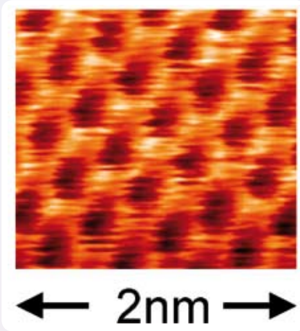
Abb. 3: Die Oberfläche von Graphit (reiner Kohlenstoff, beispielsweise verwendet als Bleistiftmine), aufgenommen mit dem Rastertunnelmikroskop. Man erkennt deutlich ein regelmäßiges Lochmuster, aufgebaut aus Kohlenstoffatomen.
